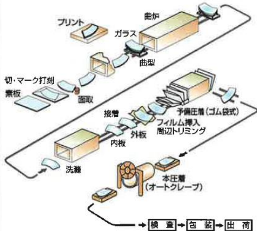
合わせガラス製造工程
