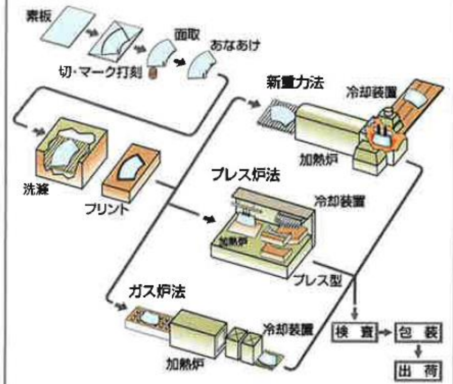
強化ガラス製造工程
